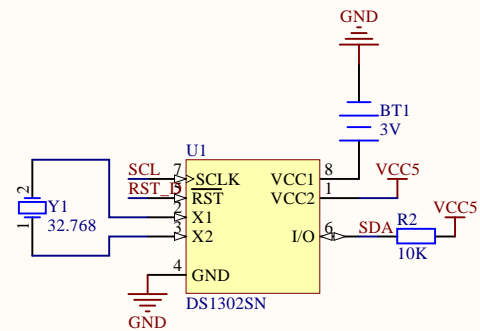
DS1302实时时钟
